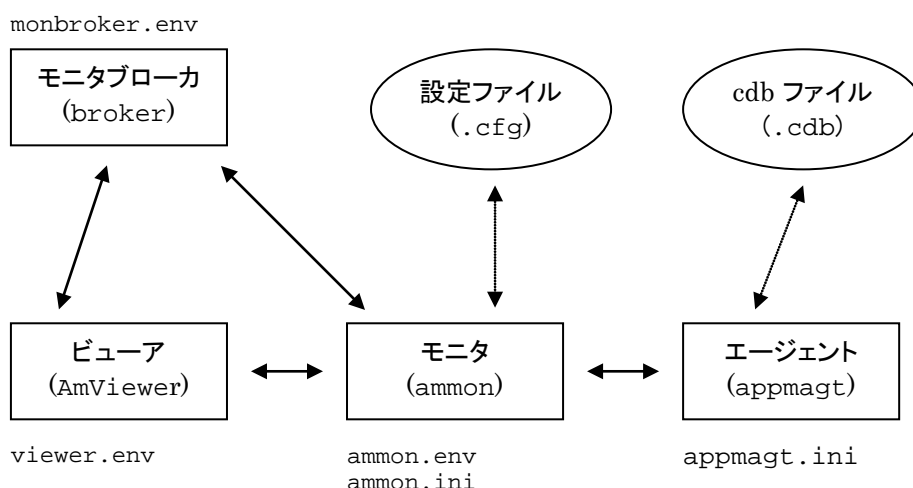
図 6.1 : チュートリアルのコポーネントとキーファイル
