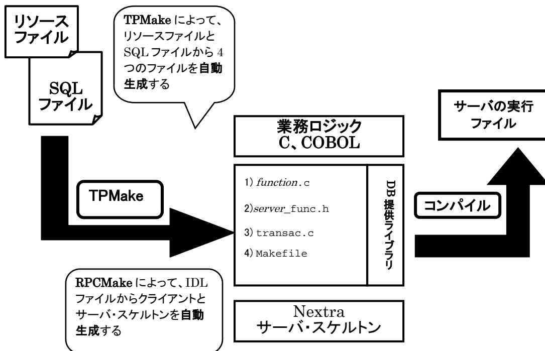
図 2.1: TPMake の使用
